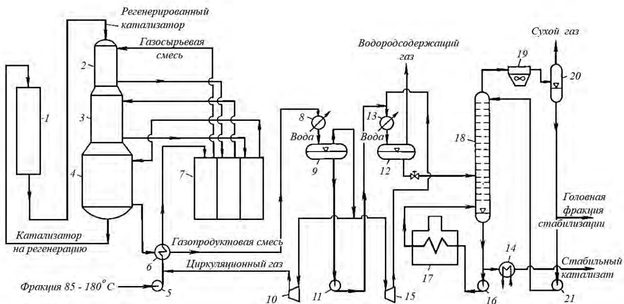
Рис. Технологическая схема установки риформинга с движущимся слоем катализатора: 1 – секция регенерации; 2 – 4 – реакторы платформинга; 5, 11, 16, 21 – насосы; 6, 14 – теплообменники; 7 – многосекционная печь; 8, 13 – холодильники; 9, 12 – газосепараторы низкого и высокого давления; 10, 15 – компрессоры; 18 – стабилизационная колонна; 17 – трубчатая печь; 19 – аппарат воздушного охлаждения; 20 – газосепаратор
